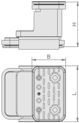
Tasarım verileri VCBL-K2 130x30x100 Q
