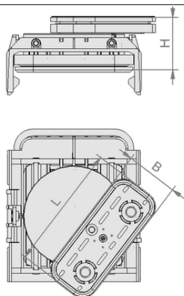
Конструктивные данные VCBL-K1 120x50x50 D-360
