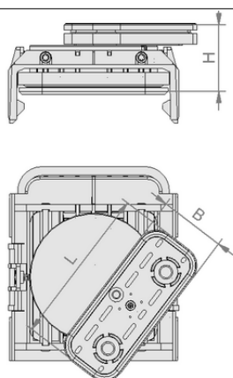
デザインデータ VCBL-K1 120x50x50 D-360
