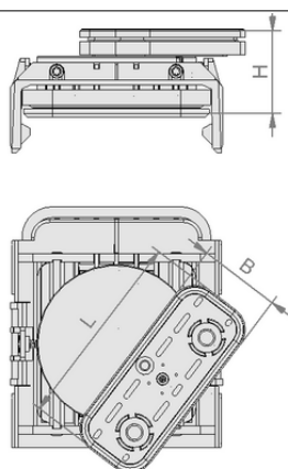
Données de construction VCBL-K1 120x50x50 D-360
