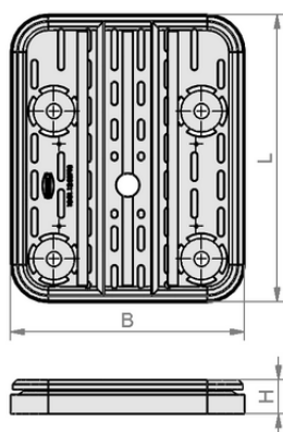
Dati di costruzione VCSP-U 140x115x16.5 VCBL-K2 TPE
