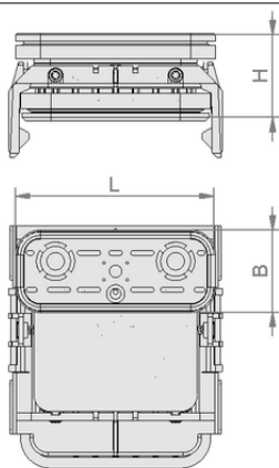
デザインデータ VCBL-K1 120x50x50 Q
