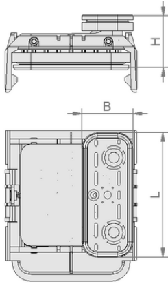
Tasarım verileri VCBL-K1 120x50x50 L
