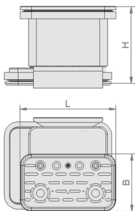
Dati di costruzione VCBL-K2 130x30x50 L
