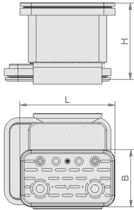
Tasarım verileri VCBL-K2 130x30x50 L
