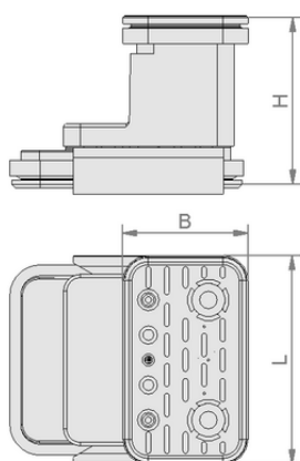
Données de construction VCBL-K2 130x30x50 Q
