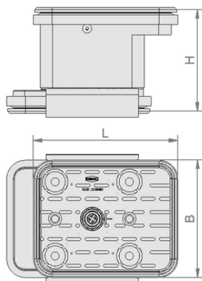
デザインデータ VCBL-K2 140x115x50
