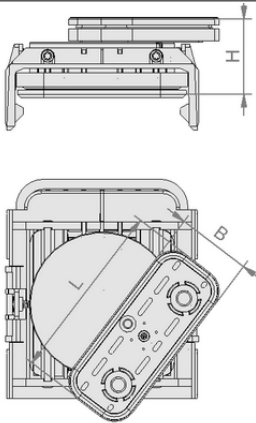
Tasarım verileri VCBL-K1 125x75x50 D-360
