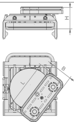
デザインデータ VCBL-K1 125x75x50 D-360
