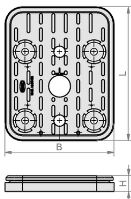
デザインデータ VCSP-O 140x115x16.5 TPE
