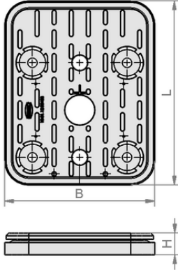
Tasarım verileri VCSP-O 140x115x16.5 TPE
