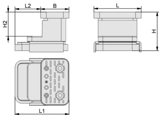
Datos de diseño VCBL-K2 125x75x100 Q
