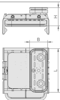
Données de construction VCBL-K1 125x75x50 L TV
