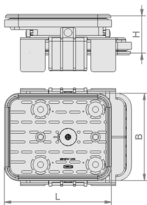
Конструктивные данные VCBL-K1 140x115x50 TV
