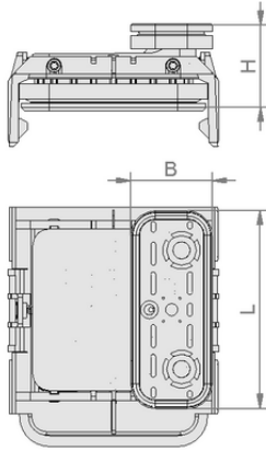
Tasarım verileri VCBL-K1 125x75x50 L
