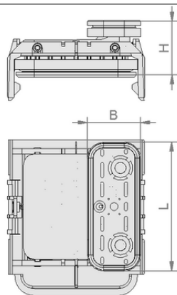
Données de construction VCBL-K1 125x75x50 L
