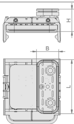
Конструктивные данные VCBL-K1 125x75x50 L
