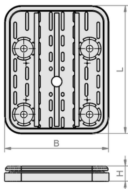
デザインデータ VCSP-U 140x115x16.5 VCBL-K1 TPE
