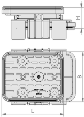
Tasarım verileri VCBL-K1 140x115x50
