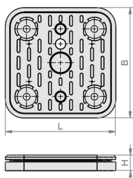
デザインデータ VCSP-U 120x120x16.5 VCBL-G TPE
