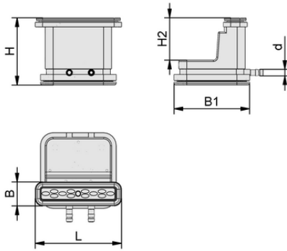
Tasarım verileri VCBL-G-K2 130x30x100 ST
