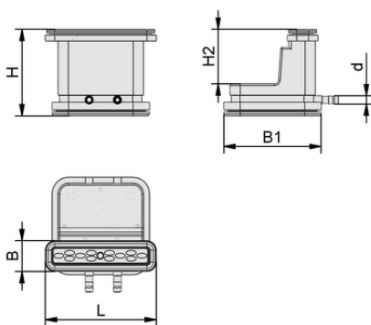
デザインデータ VCBL-G-K2 130x30x100 ST
