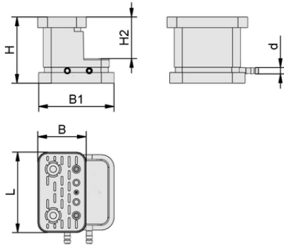
Tasarım verileri VCBL-G-K2 125x75x100 ST
