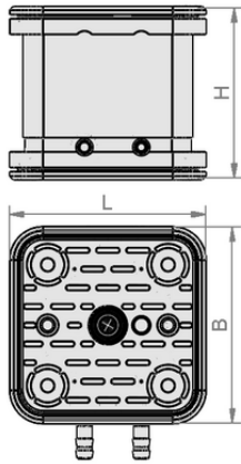
Tasarım verileri VCBL-G-K2 120x120x100 ST+AS
