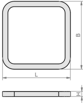
Tasarım verileri VCDR 120x120x8 BL
