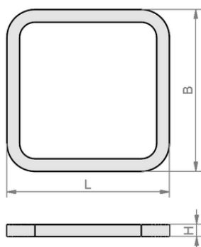
デザインデータ VCDR 120x120x8 BL
