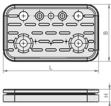
デザインデータ VCSP-O 120x50x15.5 TPE
