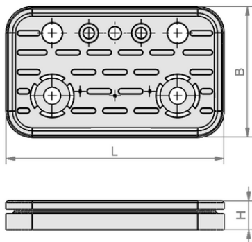
デザインデータ VCSP-O 125x75x16.5 TPE
