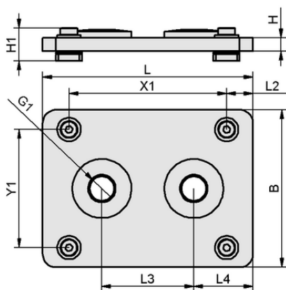
Konstruktionsdaten FLAN-PL 160x120x10 FMHD
