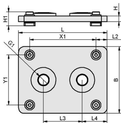
Dati di costruzione FLAN-PL 160x120x10 FMHD
