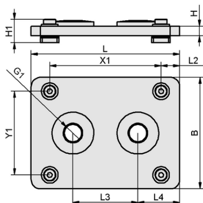
デザインデータ FLAN-PL 160x120x10 FMHD
