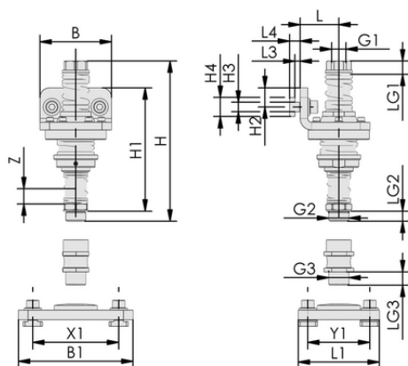
デザインデータ FST-FLEX 75 HD1 G1/2-AG G3/8-IG
