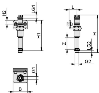
Datos de diseño FST-STARR 75 HD1 G1/2-AG G3/8-IG
