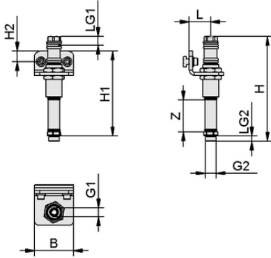
Tasarım verileri FST-STARR 50 HD1 G1/2-AG G3/8-IG
