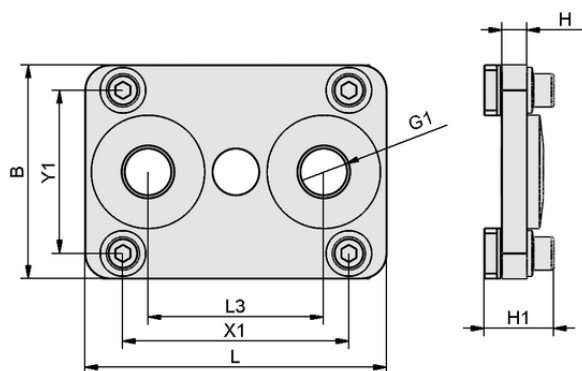
Datos de diseño FLAN-PL 120x85x10 ST FLGR
