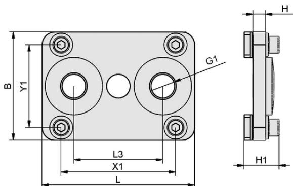
Konstruktionsdaten FLAN-PL 120x85x10 ST FLGR
