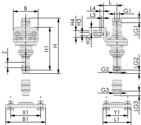
Tasarım verileri FST-FLEX 50 HD1 G1/2-AG G3/8-IG
