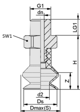
デザインデータ FSGA 33 NK-45 G1/4-AG FP80
