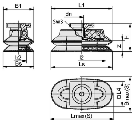
Dati di costruzione SAOXB 40x20 ED-85 RA MOD
