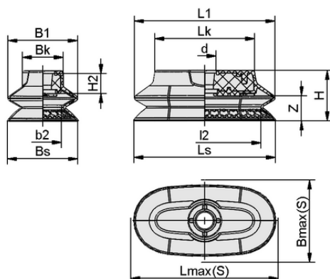
デザインデータ SAOXB 110x55 ED-85 SC043
