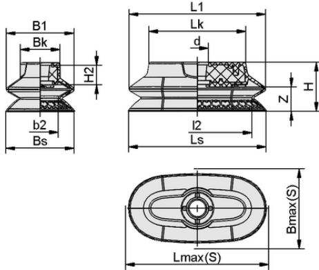
Tasarım verileri SAOXB 60x30 ED-85 SC043
