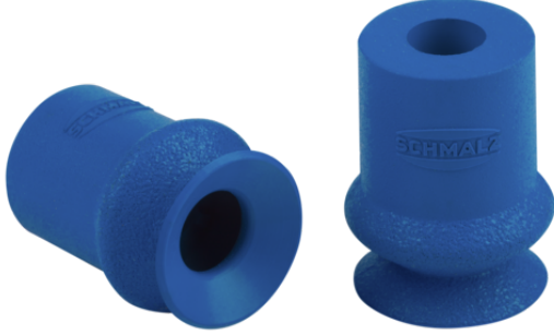
FGA 12 HT1-60 N016
