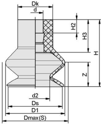
Tasarım verileri FGA 12 HT1-60 N016
