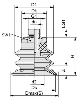
デザインデータ SDC2 50 PU 30/60 G1/4-AG
