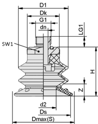
Datos de diseño SDC2 50 PU 30/60 G1/4-AG
