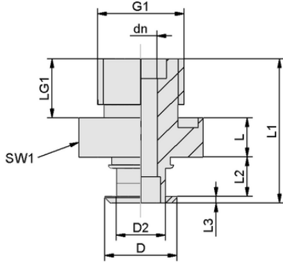
Tasarım verileri SA-NIP N044 G1/4-AG DN800
