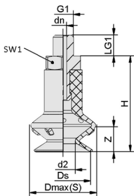
Datos de diseño FSGA 8 SI-HD-65 M3-AG
